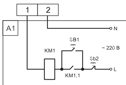
Подключение блока управления (A1)
