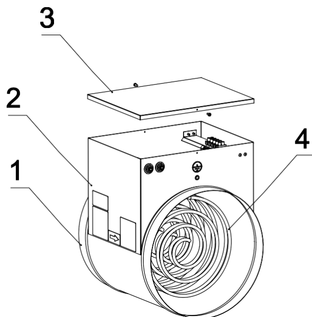
1 - корпус; 2 - клеммная коробка; 3 - крышка клеммной коробки; 4 - ТЭН Рисунок 1.1 - Состав электронагревателя ЭНК
